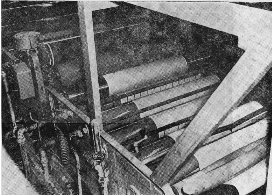
B. चेनलेस मर्सराइझिंग मशीन (लाय इंप्रेगनेशन सेक्शन)
