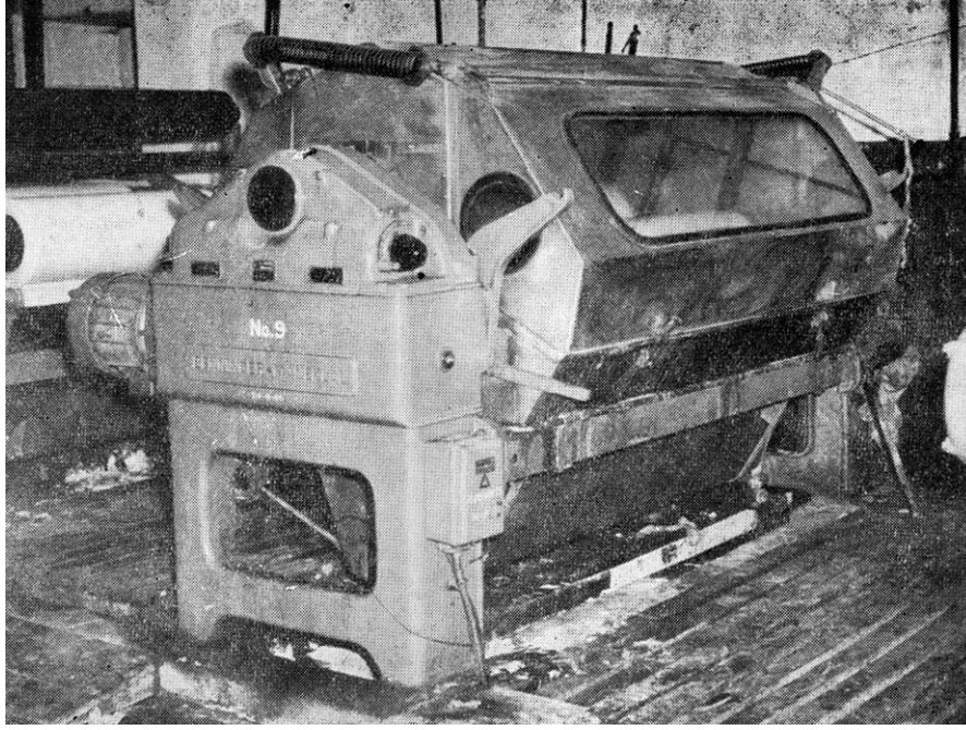
F. ऑटोमेटिक डायिंग जिगर
