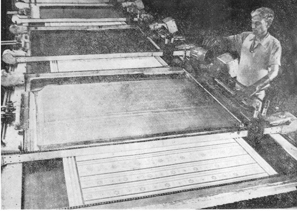
H. साडीचा पदरही छापण्याची सोय असलेले ऑटोमेटिक फ्लॅटबेड स्क्रीन प्रिंटिंग मशीन
