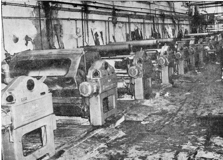
G. स्वयंचलित जिगर यंत्रांची रांग
