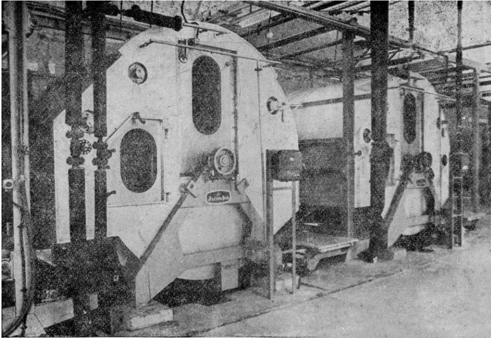
D. थर्मो – रिअॅक्शन चेंबर (जम्बो – टाईप)
