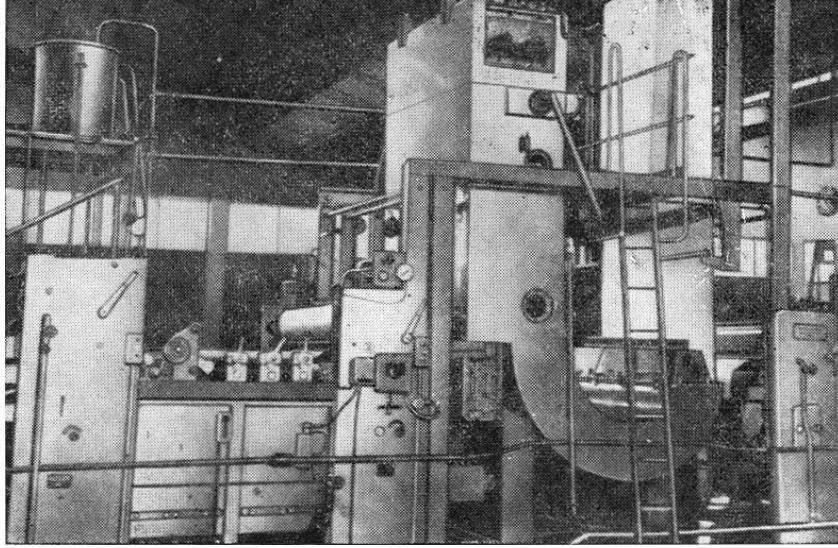
C. कंटिन्यूअस रोप ब्लीचिंग प्लॅट (जे बॉक्स)
